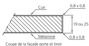
Coupe de la façade porte et tiroir
