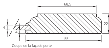
Coupe de la façade porte
