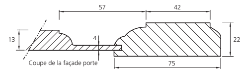
Coupe de la façade porte
