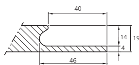
Coupe de la façade porte et tiroir (bord haut ou bas)
