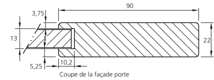
Coupe de la façade porte
