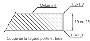
Coupe de la façade porte et tiroir
