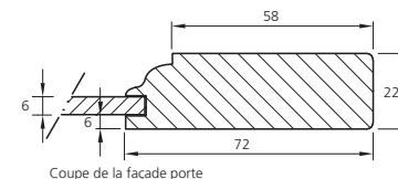
Coupe de la façade porte
