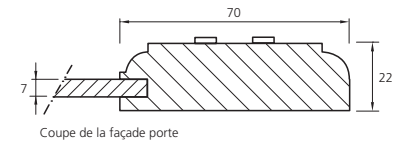
Coupe de la façade porte
